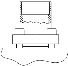
FLANGIA QUADRA/ SQUARE FLANGE
